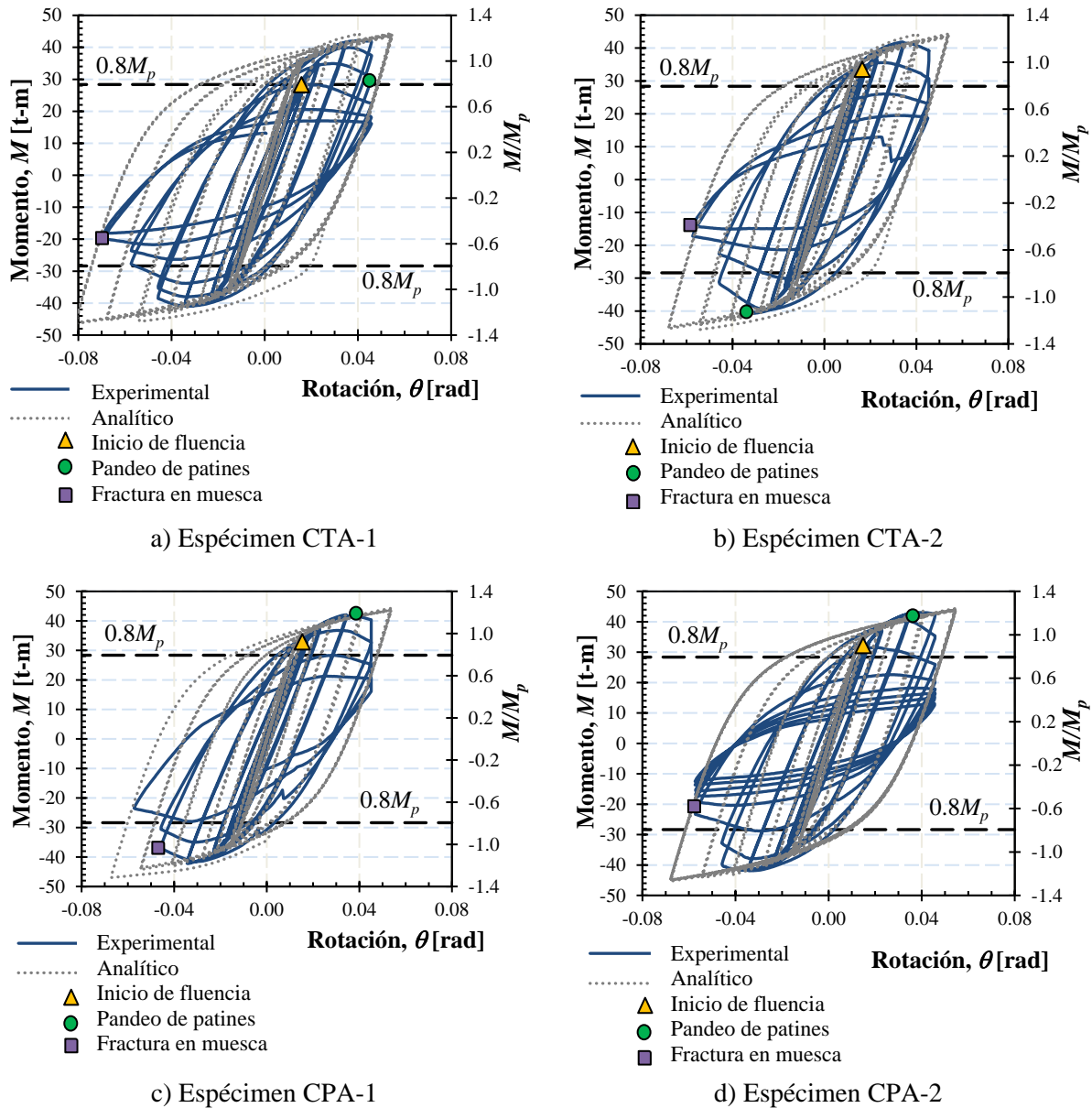
Figura 7. Comparación de resultados del análisis ante carga cíclica
