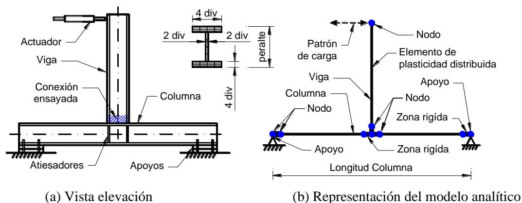
Figura 8. Características del modelo en estudio
