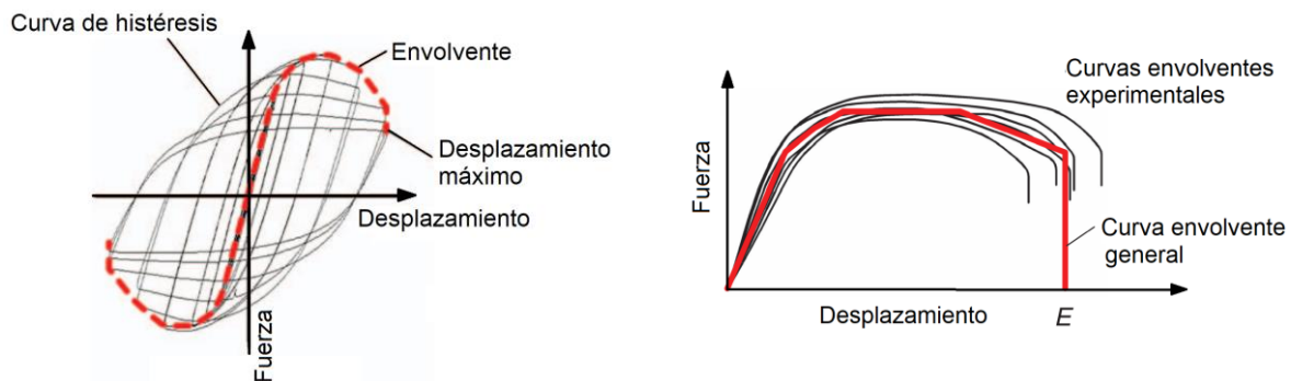
a) Curva envolvente de una prueba experimental b) Construcción de la curva envolvente general
