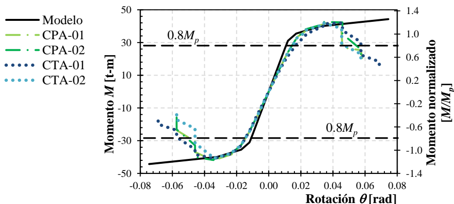
Figura 9. Comparación de curvas de capacidad y la envolvente de la respuesta experimental
