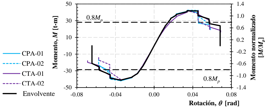
Figura 12. Curva de columna derivada de envolventes de datos de prueba experimentales
