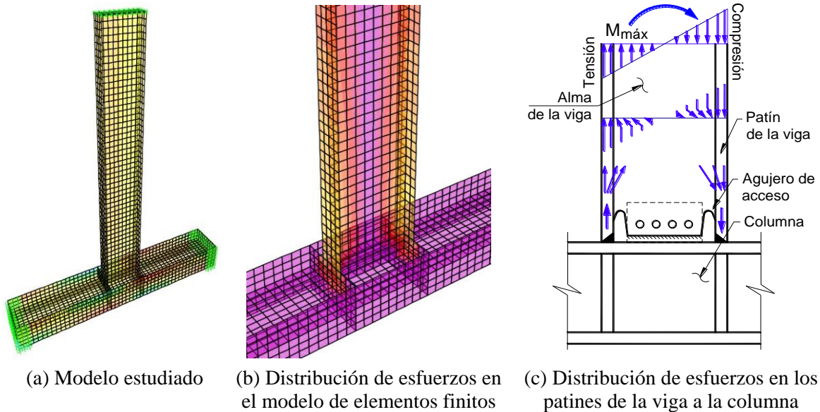
Figura 5. Modelo analítico y distribución de tensiones críticas
