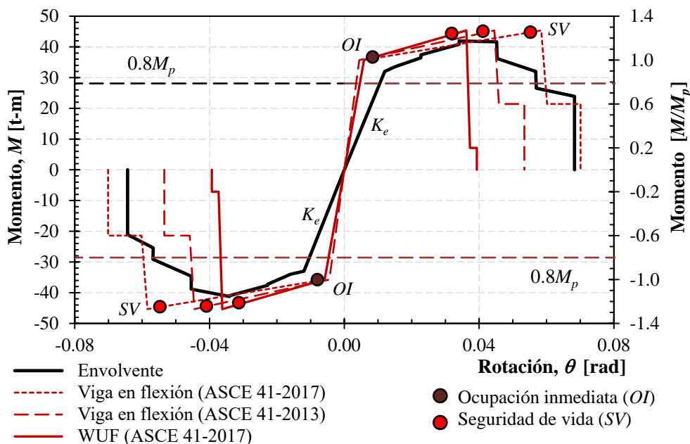
Figura 13. Curvas idealizadas de fuerza-desplazamiento y curva envolvente
