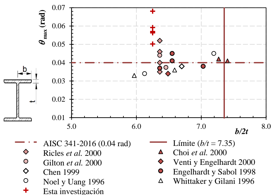
Figura 4. Rotación plástica en función de la esbeltez del patín de la viga
