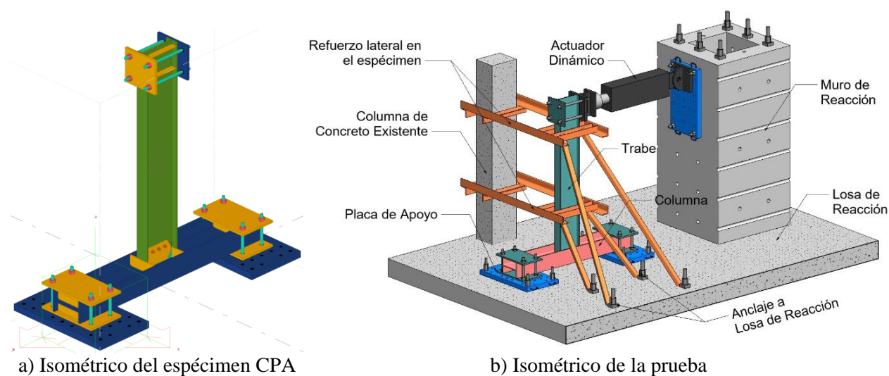
Figura 2. Configuración de la prueba experimental
