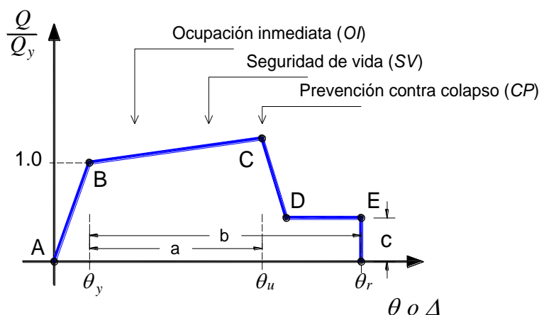
Figura 11. Curva fuerza-deformación generalizada para elementos de acero
